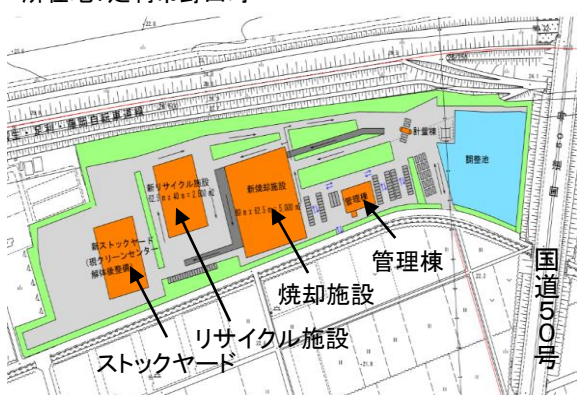
新クリーンセンター施設配置イメージ図 所在地:足利市野田町
